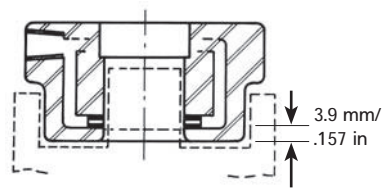
Snout Type
